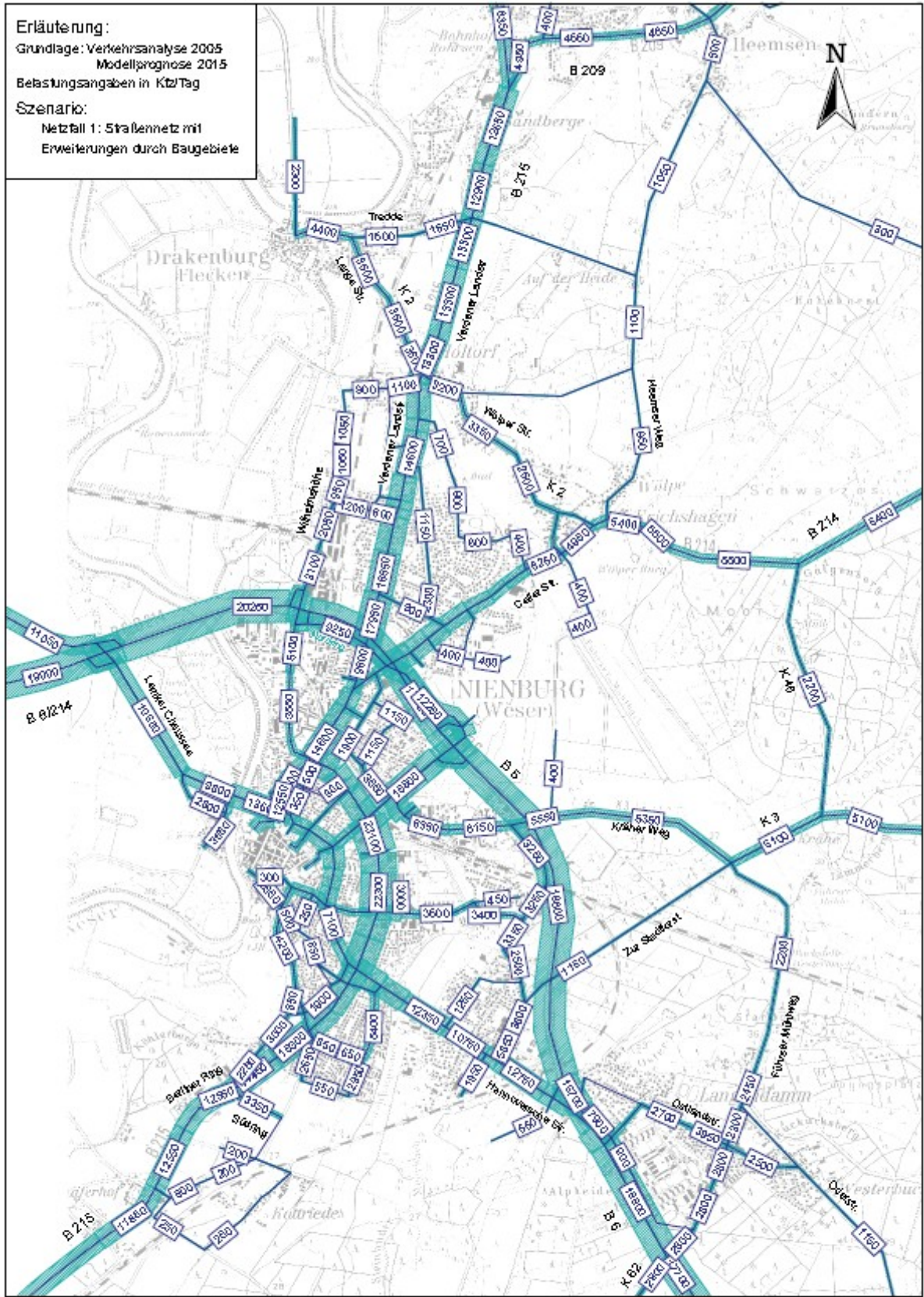
PROGNOSEBELASTUNGEN 2015 IM VORHANDENEN STRASSENNETZ IM RAUM NIENBURG / HEEMSEN - NETZFALL 1 - AUSSENBEREICH
