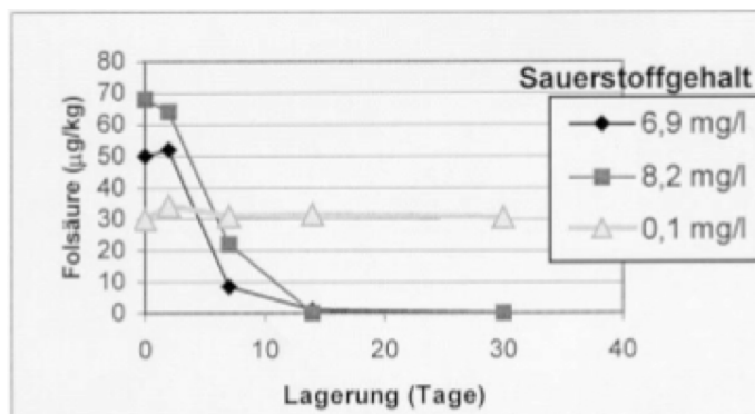
Abb. 8: Verhalten der Folsäure während der Lagerung von UHT-Milch bei RT in Abhängigkeit vom Sauerstoffgehalt (16).
