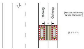
Regelplan B II / 1.1
