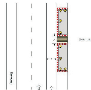
Regelplan B II / 1.5
