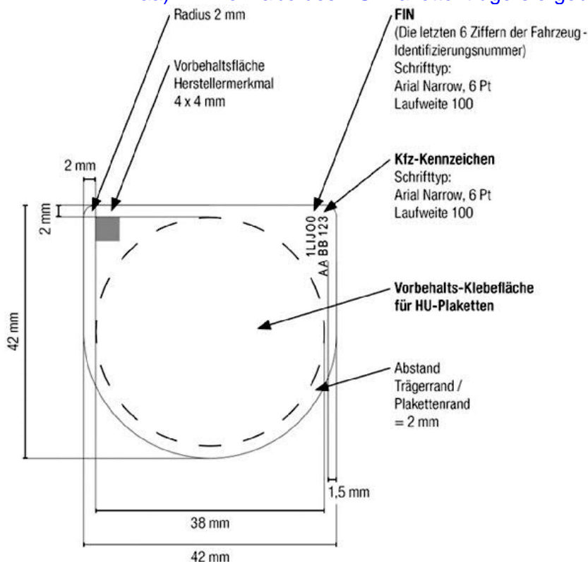
Abbildung 5: Bemaßung des HU-Plakettenträgers
